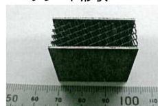
メッシュ形状
